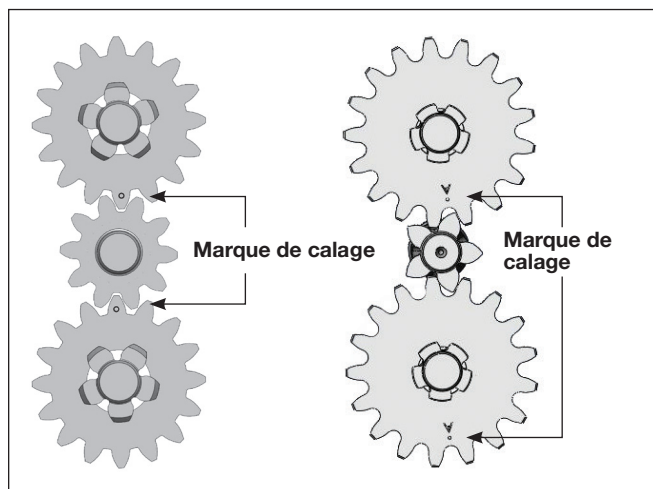
Figure 10 - Synchronisation des vitesses (0.75, 1 et 1.5 Tonne) Figure 11 - Synchronisation des vitesses (3 et 6 Tonne)
