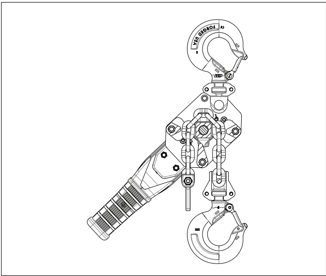
Installation en chaîne à passage unique (0.75 - 3 Tonne)
