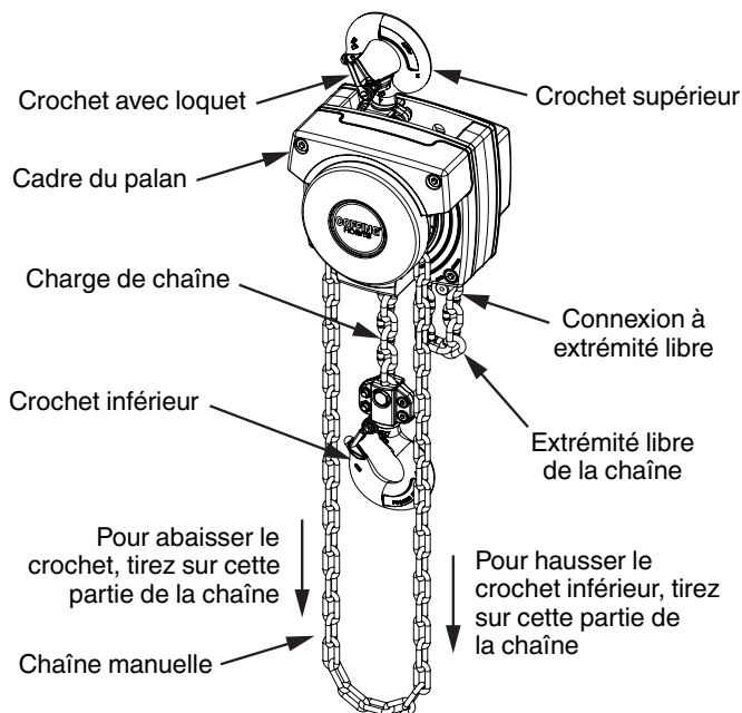
Figure 2 - Composantes principales du palan Coffing® LHH-NC
