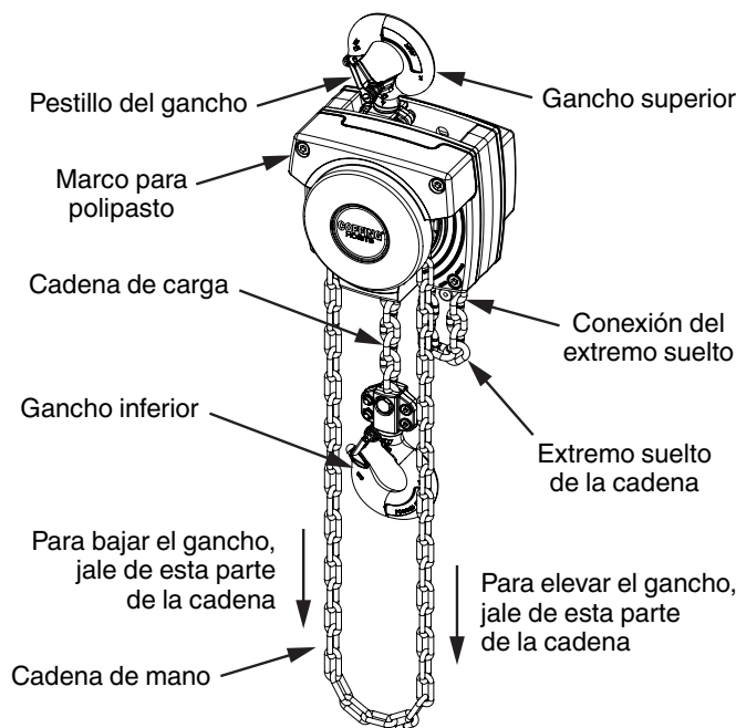
Figura 2 - Piezas principales del polipasto Coffing® LHH-NC
