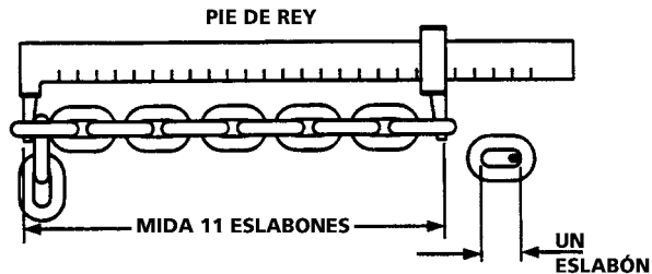
Figura 5 - Inspección de la cadena
