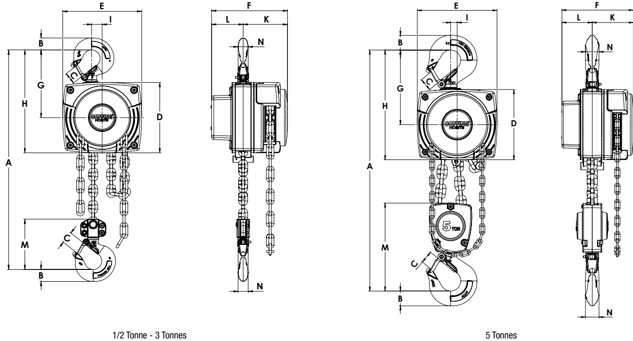
Figure 1 – Spécifications & Dimensions
